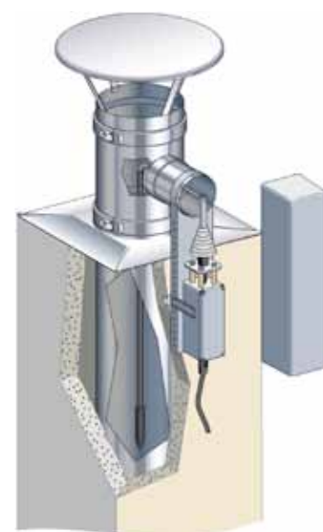
sortie de toit TOP CLEAN pour conduit maçonné
