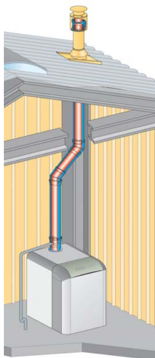
Figure 1 – Schéma de principe avec terminal vertical C 33
