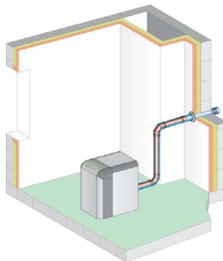
Figure 2 – Schéma de principe avec terminal horizontal C 13
