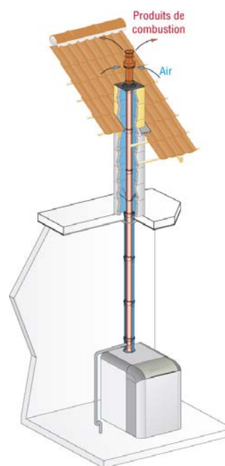
Figure 3b - Réutilisation d'un conduit existant départ plafond
